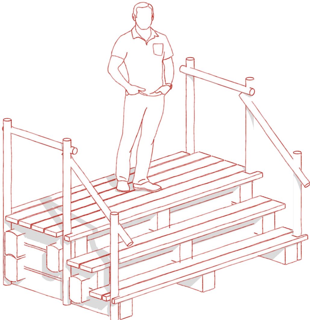
Persp Skala 1:20
